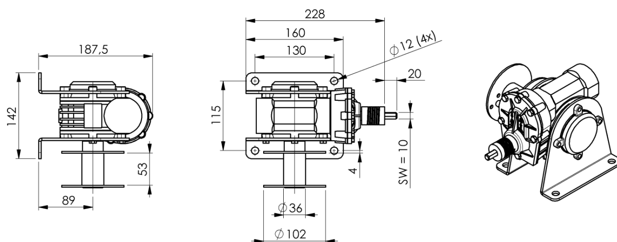
Dimensioni dell'organo per il montaggio a pavimento (console).
