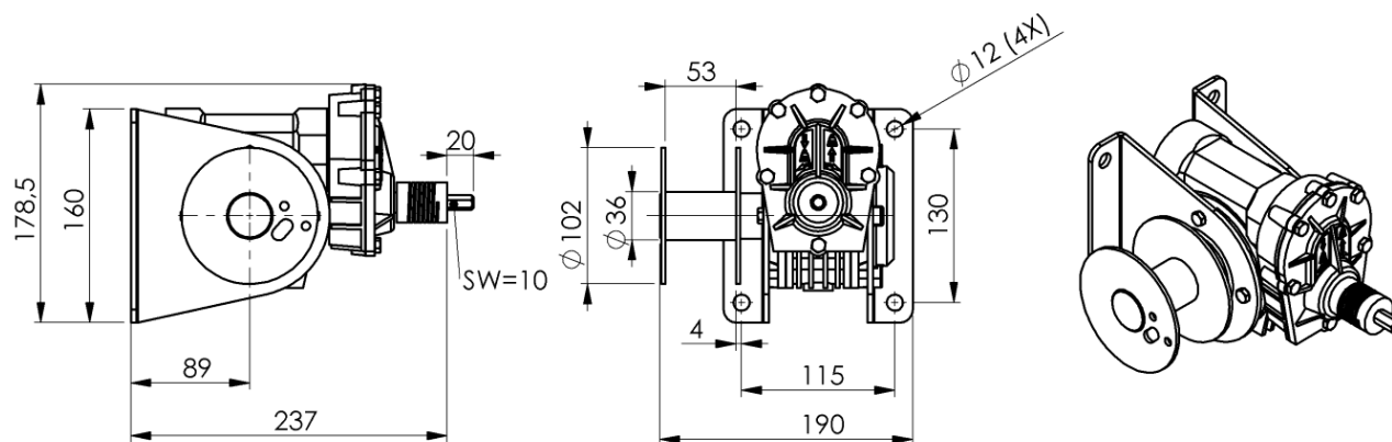
Dimensioni dell'organo per il montaggio a pavimento (console).
